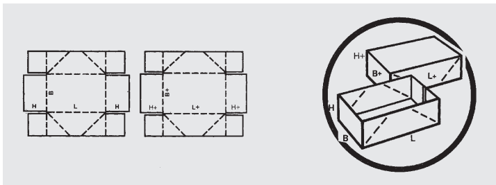
fefco 0303 Stülpkarton gestanz mit 4-Punkt-Klebung Außenfaltung
