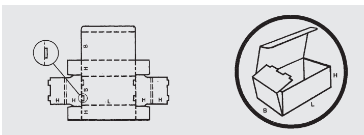
fefco 0421 Wellkartonsschachtel gestanz, stirnseitig eingeschlagen, mit anhängendem Deckel
