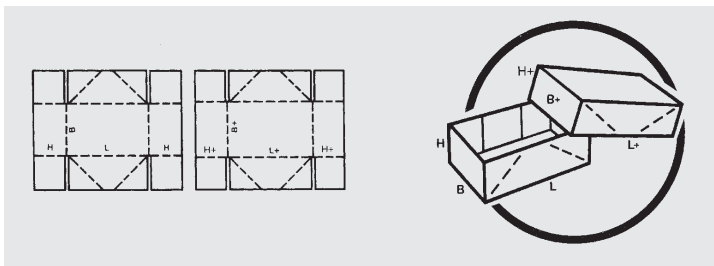
fefco 0304 Stülpkarton, gestanz mit 4-Punkt-Klebung, Innenfaltung
