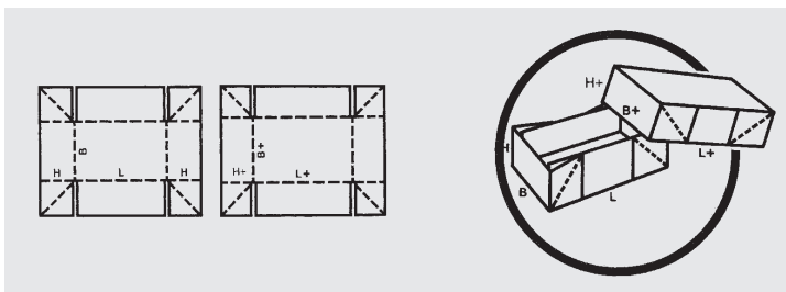
fefco 0308 Stülpkarton, gestanz mit 4-Punkt-Klebung, Außenklebung
