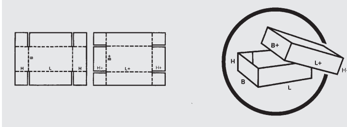
Fefco 301 Stülpkarton, geheftet
