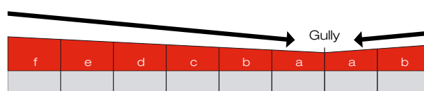
Verlegeschema A: mit flapor-Gefälledämmplatten
