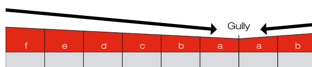
Verlegeschema A: mit flapor plus-Gefälledämmplatten
